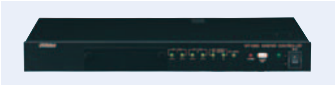
マスターコントローラー WT-M60 ●電源:AC 100 V、50 Hz / 60 Hz ●消費電力:21W ●モニター出力:×2、φ6.3 複式フォノジャック、0 dBs ±2 dBs、100 Ω、電子平衡 ●外部入力:×2、端子板、—20 dBs、10 k Ω、トランス平衡 ●外形寸法:幅420 mm ×高さ44 mm ×奥行280 mm (突起物含まず) ●質量:3.0 kg
