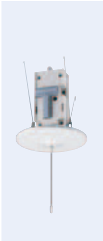
マスタートランシーバー WT-T60 ●空中線電力:10mW●アンテナ:1/4λ ホイップアンテナ ●電源:DC15VまたはDC12V●外形寸法:φ150mm×高さ160mm●質量:0.285kg (取付金具を除く)
