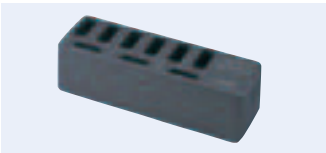
チャージャー WD-C12 ●電源:AC 100 V、50 Hz / 60 Hz ●消費電力:42 VA ●出力:DC 4.2 V 400 mA (9 回路) ●同時充電可能数:最大6台 (WT- TR60)、最大3台 (専用バッテリー) ●充電時間:最大約4時間 ●外形寸法:幅360 mm ×高さ107 mm ×奥行120 mm ●質量:1.0 kg
