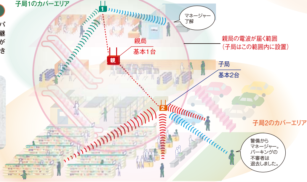
屋内に設置した中継局のイメージ 壁掛け時計を取り付けるのと変わらない手軽さで設置できます。
